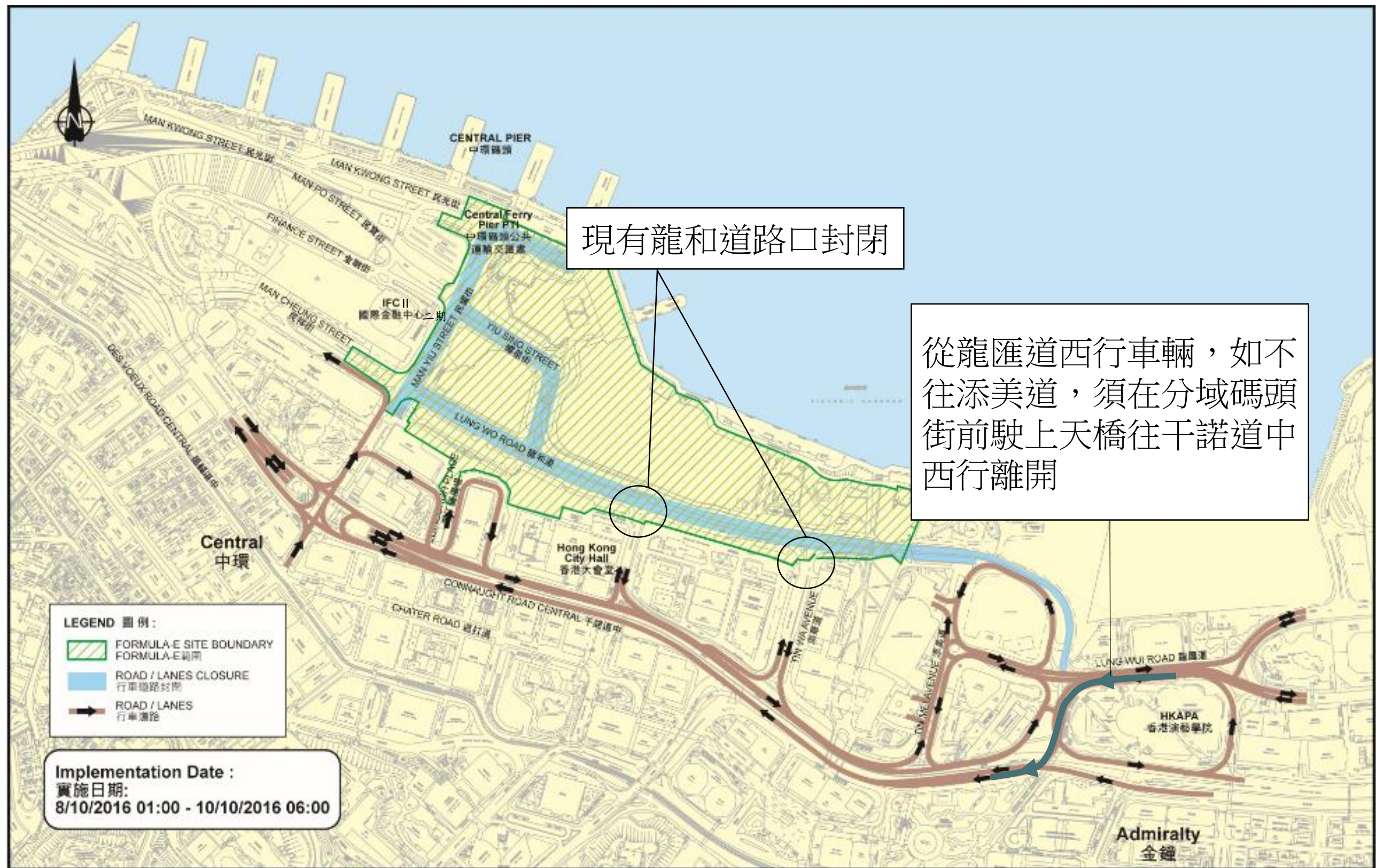
圖 3.3 賽事期間的臨時行車路線 (賽區以東)
